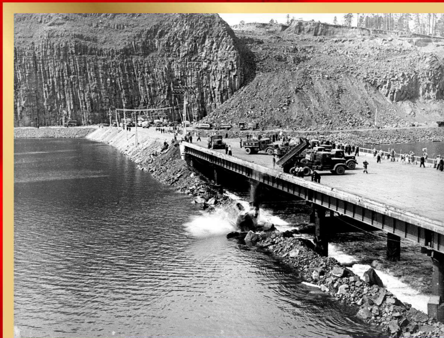
Перекрытие левобережной части р. Ангары. 1959 год.
