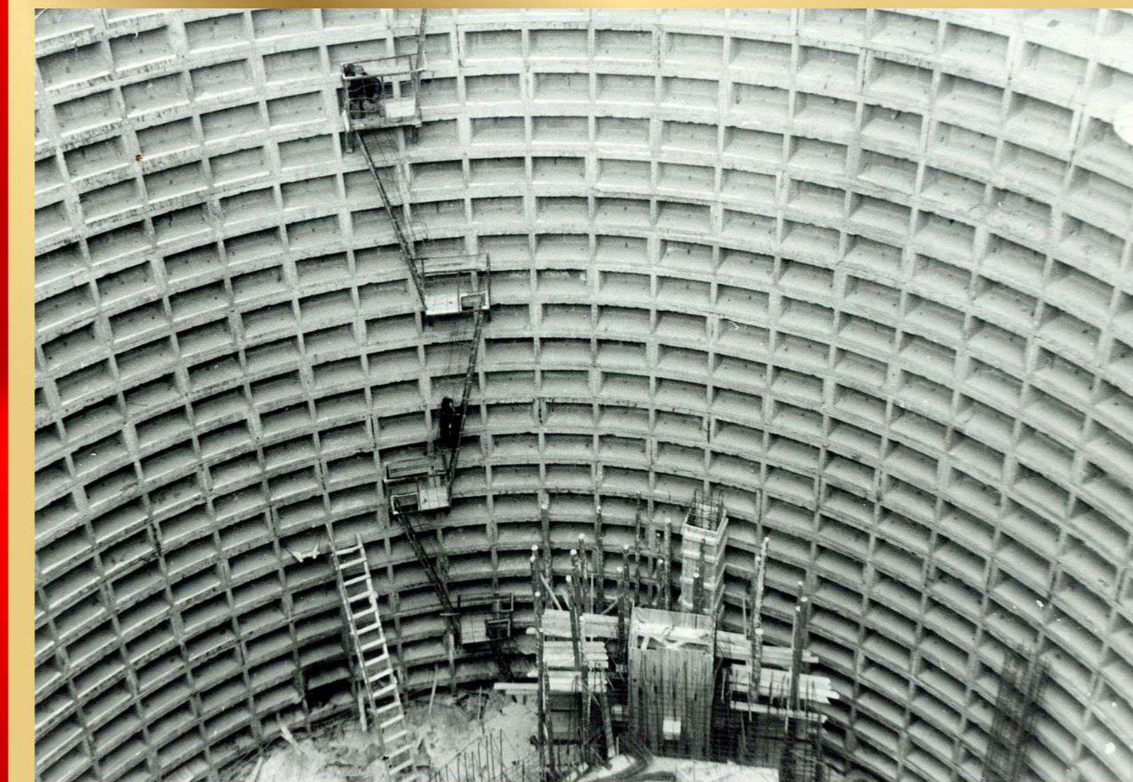
Монтажные работы на обогатительной фабрике. Иркутская область, посёлок Железногорск, 1963 год.
