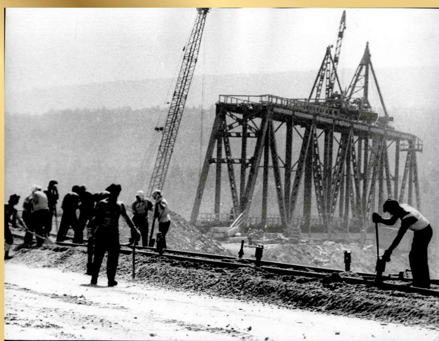
Первые метры БАМа. Работает Мостоотряд-45. Посёлок Магистральный.
